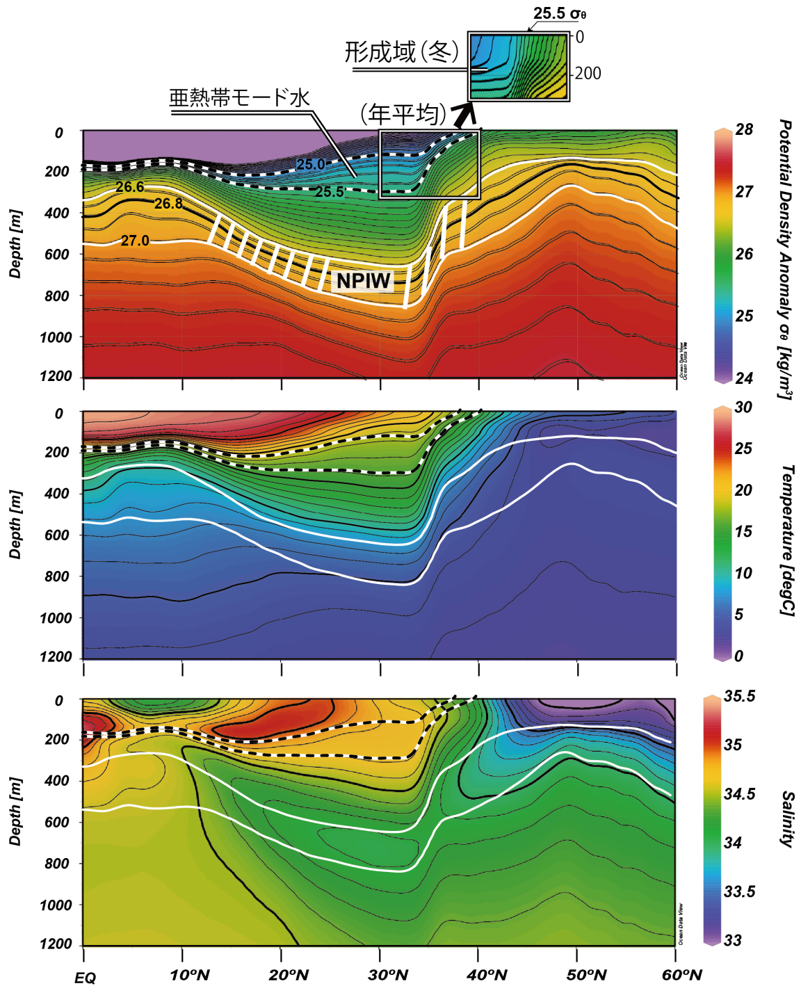
北太平洋における、 年平均 の密度アノマリ（上）、水温（中）、塩分（下）の南北鉛直断面図。亜熱帯モード水の範囲を白黒破線、北太平洋中層水（NPIW）を太白線枠内で表した。冬（1-3月平均）の30-40°N、0-300 m範囲の密度アノマリ拡大図を最上段。
