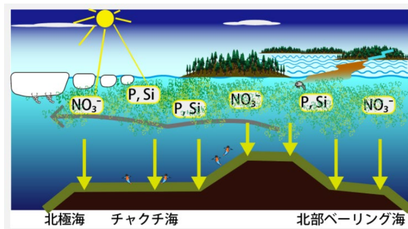
図 海水融解後に起こる植物プランクトンの大増殖（ブルーム）
