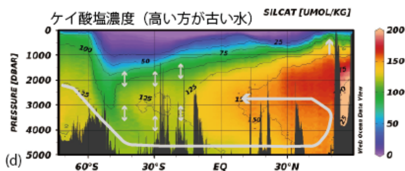
図（つづき） 南北太平洋におけるケイ酸塩濃度の鉛直断面
