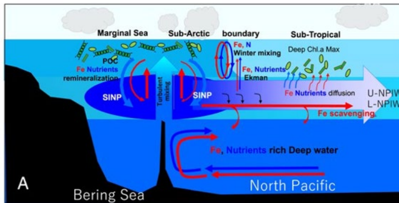
図 北太平洋の深層-中層循環 (Nishioka et al., PNAS, 2020: doi: 10.1073/pnas.2000658117, Fig4)
