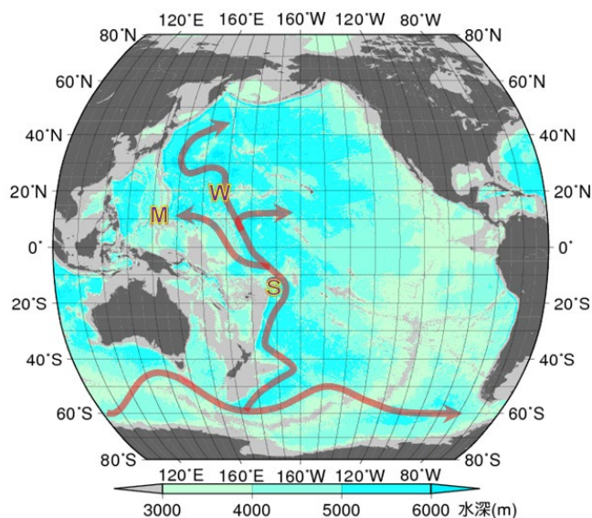
図 太平洋を流れる南極底層水の主な経路（気象庁ホームページの海洋の総合診断表より引用） 海底地形に沿って底層水が大河のようにウネウネ流れている。
