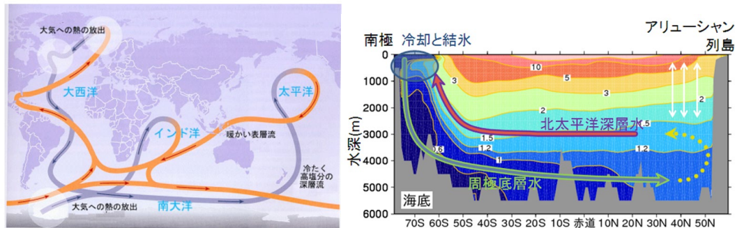
左図 ベルトコンベヤーモデル（気象庁 HP）
