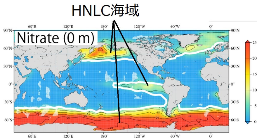
図 HNLC 海域：表層で硝酸塩が年間を通して余っている。
