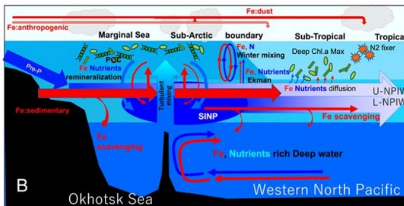
図 北太平洋の深層-中層循環
