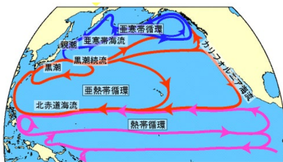
左図 北太平洋の海洋循環（気象庁 HP）
