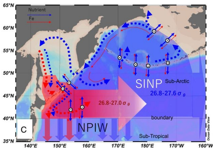
図 北太平洋の深層-中層循環（Nishioka et al. 2020） つづき
