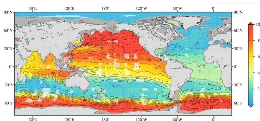
図 酸素極小層(750m)の \text{Si}(\text{OH})_4 濃度の分布
