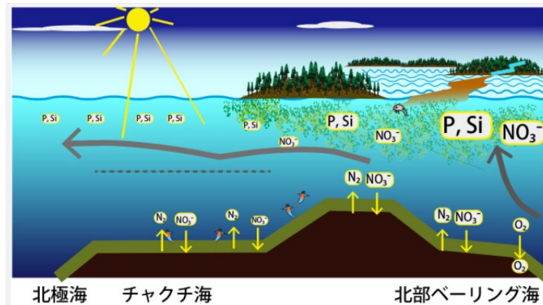
図 北部ベーリング海とチャクチ海の陸棚上で硝酸還元が起こる様子
