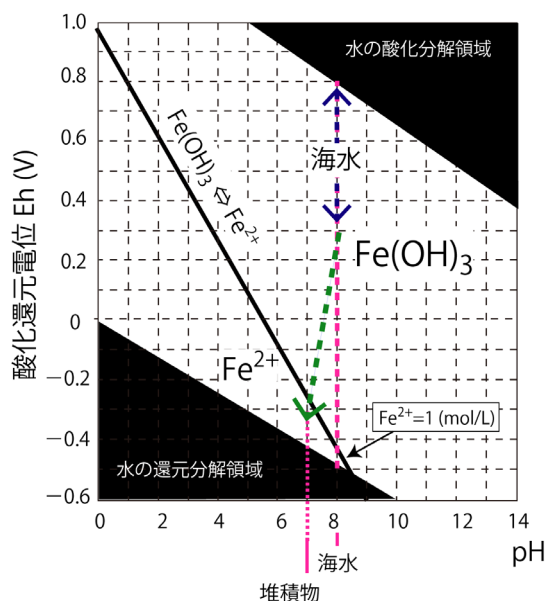
図 鉄の存在状態（ pH と酸化還元電位）のプールベ図
