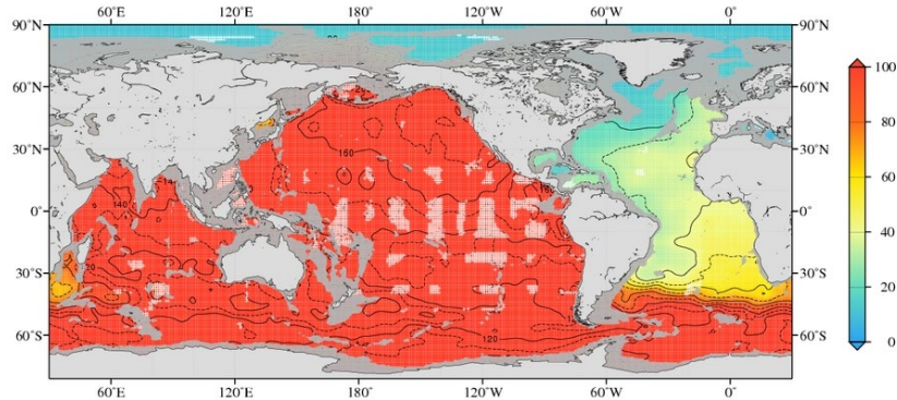
深層(3000m)の \text{Si(OH)}_4 濃度の分布
