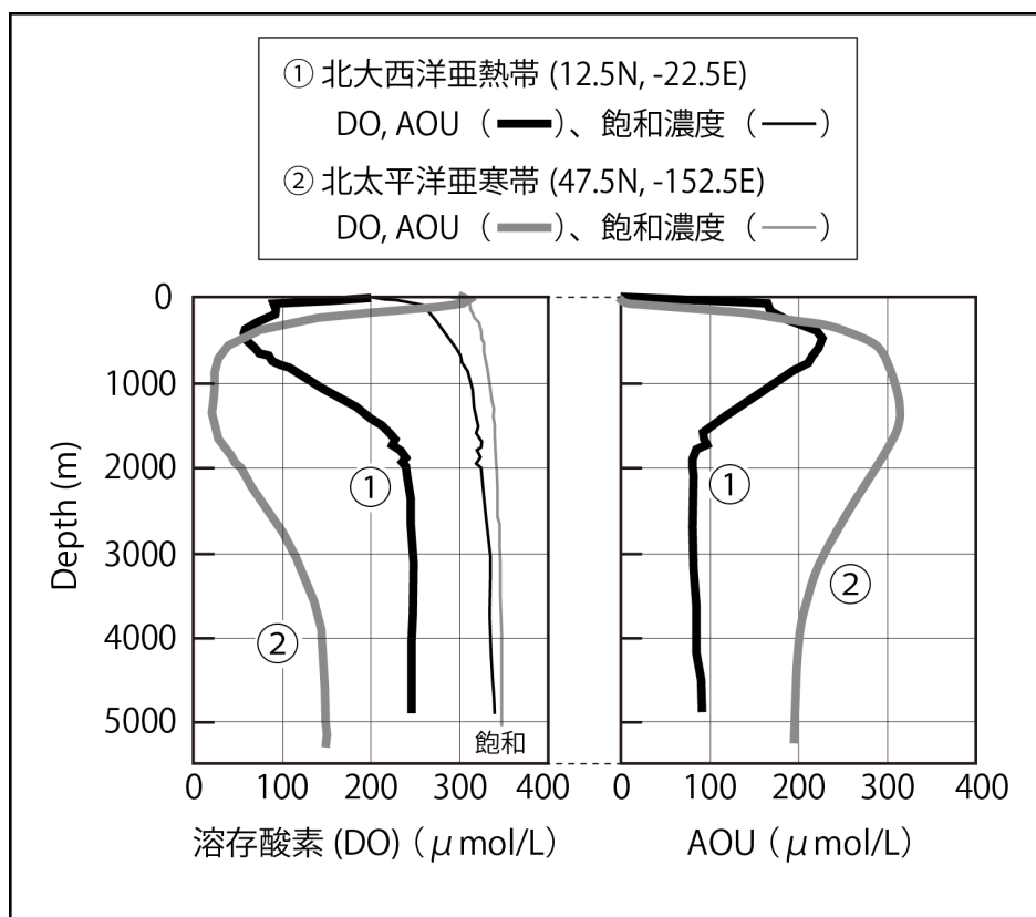
図 北大西洋亜熱帯（アフリカ大陸に近い所で生物生産性が高い）と北太平洋亜寒帯における溶存酸素（DO）とみかけの酸素消費量（AOU）の鉛直分布
