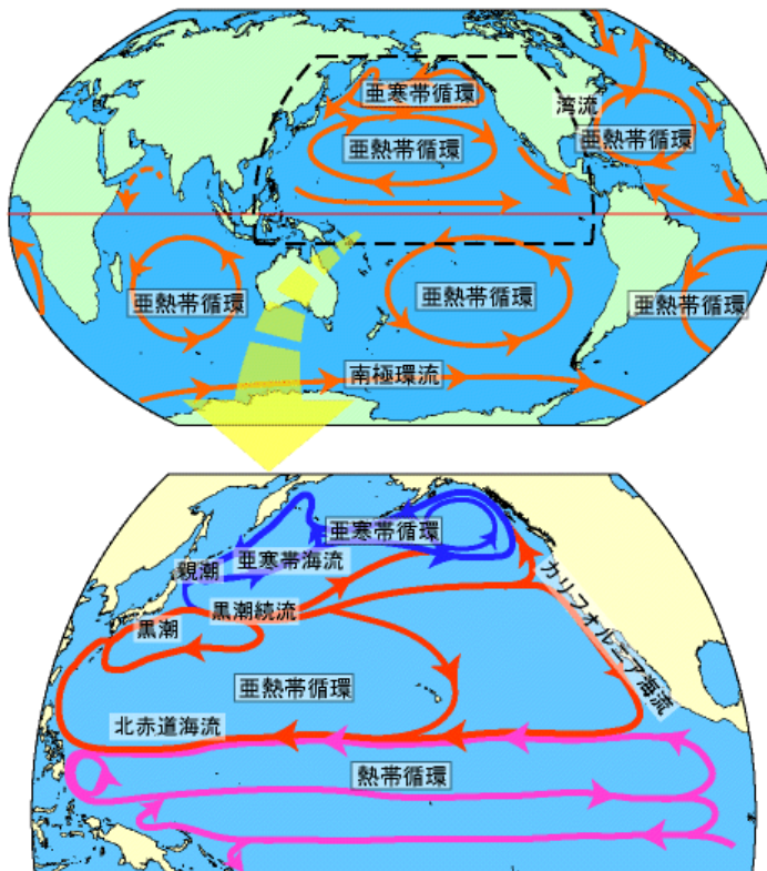
海洋の循環の模式図（気象庁 HP より）
